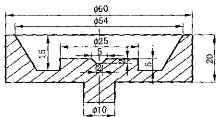
图2 下夹具示意图
